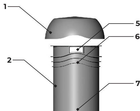
Podstawy przejściowe do blachodachówek i blachy modułowej.
